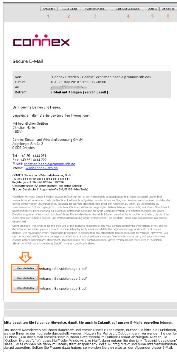
Abbildung 3: Entschlüsselte E-Mail
